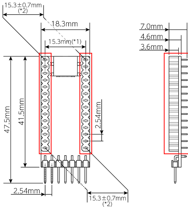
ピンソケット変更前の外形図（2022 年 12 月の以前出荷分）
