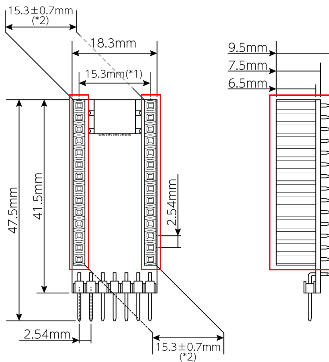
ピンソケット変更後の外形図（2023 年 1 月以降の出荷分）
